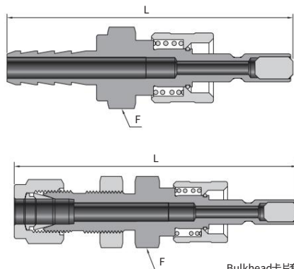
Bulkhead卡片套管接頭
