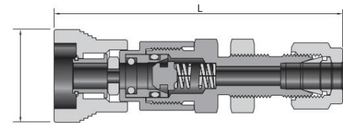
Bulkhead卡套管
