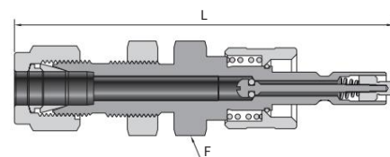
Bulkhead卡套管
