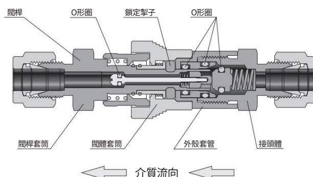
雙端關斷(DESO)
