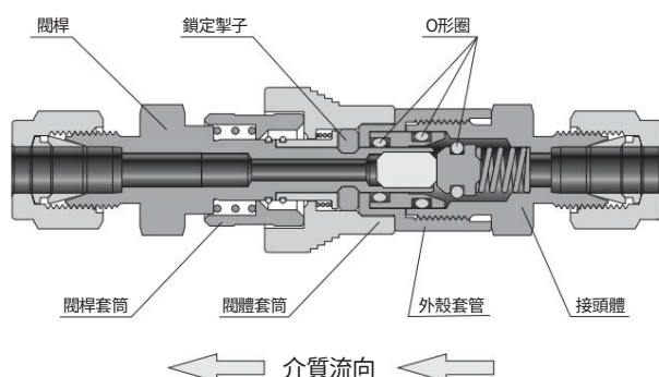
單端關斷(SES0)
